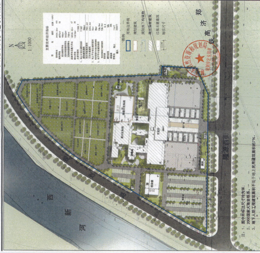
聊城市殡葬服务中心火化车间扩建项目规划总平面图
